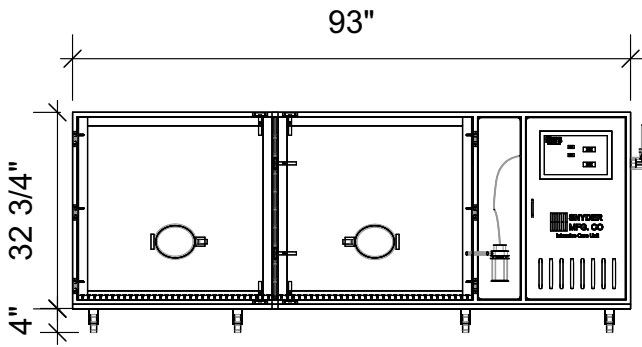
1 ICU 2 door 2100 custom 93" Scale: 3/8" = 1'-0"
