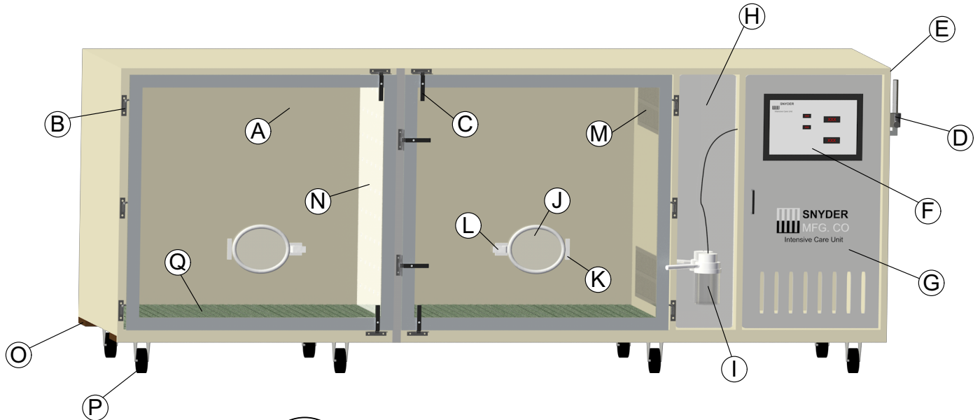
2 ICU 2 door custom 93" Scale: 3/4" = 1'-0"
